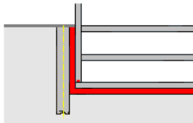
Grundwasserabdichtung Waterproofing below groundwater table
